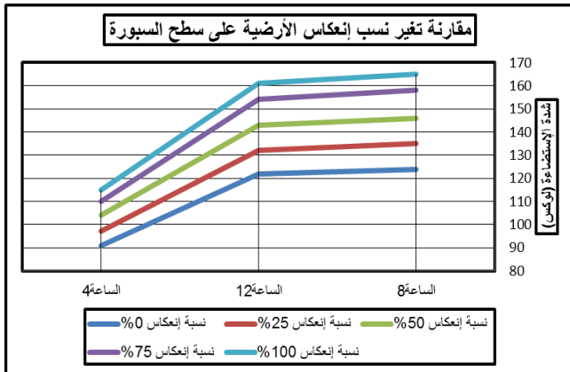
شكل (21): تأثير تغير نسب انعكاس الأرضية على سطح سبورة الفصل مع ثبات نسب انعكاس السقف والحوائط (0%)
